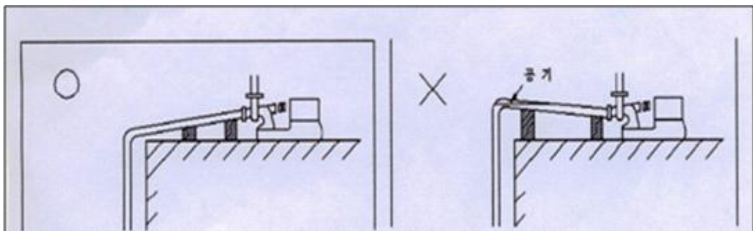
그림 1-4. 흡입배관 설치 방법
